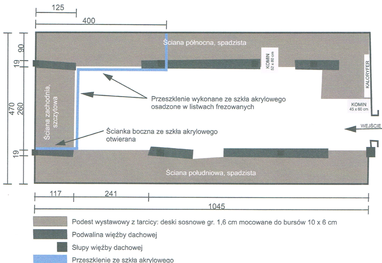
Rysunek 3 Przeszklenie, rzut poziomy
