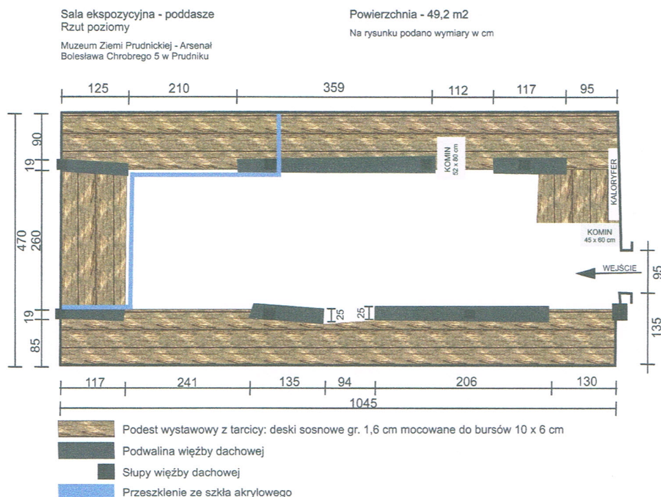
Rysunek 1 Podest wystawienniczy
